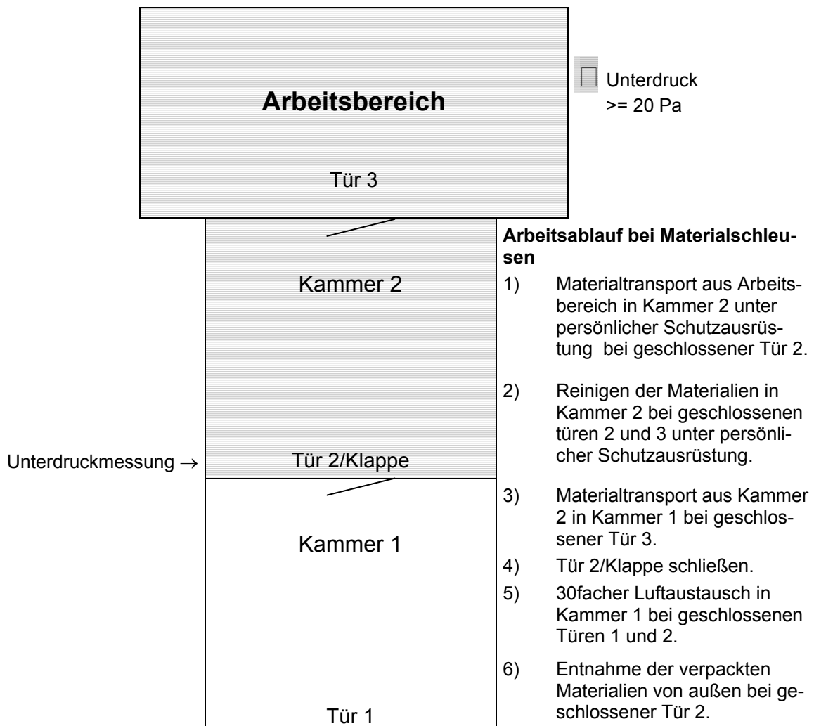
Abb. 2: Materialschleuse (Prinzipskizze)
