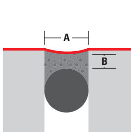
Richtig dimensionierte Fuge A:B = 2:1 Dimension A, B mind. 6 mm
