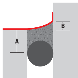
Richtig ausgeführter Winkelanschluss Dimension A, B mind. 6 mm
